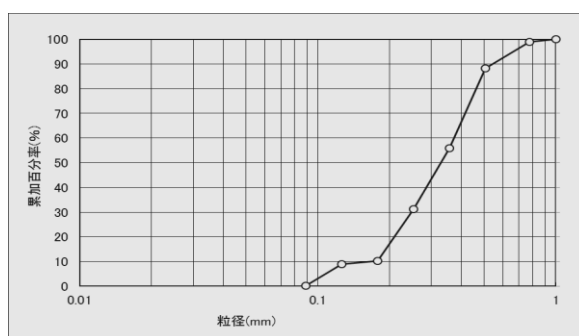
図-1 粒度分布図
