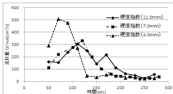
図-3 流砂量の時間変化
