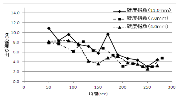
図-5 土砂濃度の時間変化
