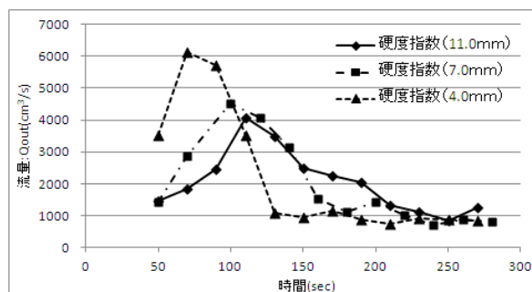
図-2 流量の時間変化
