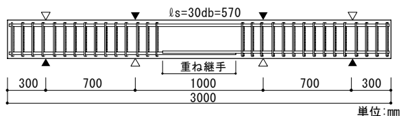
図-4 試験体形状
