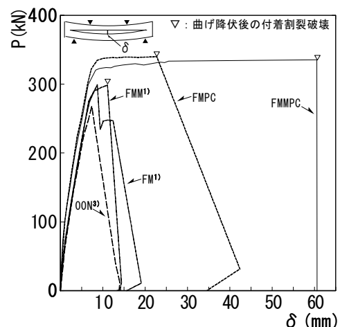
図-7 荷重-変位曲線(包絡線)
