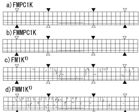
図-6 乾燥収縮ひび割れの発生状況
