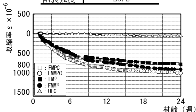
図-5 長さ変化試験体の乾燥収縮率
