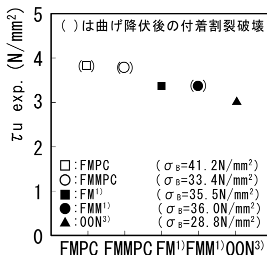
図-8 付着割裂強度
