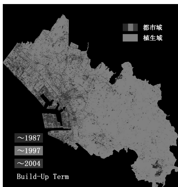
図-3 NDBI ベースの時系列的 BA 抽出画像
