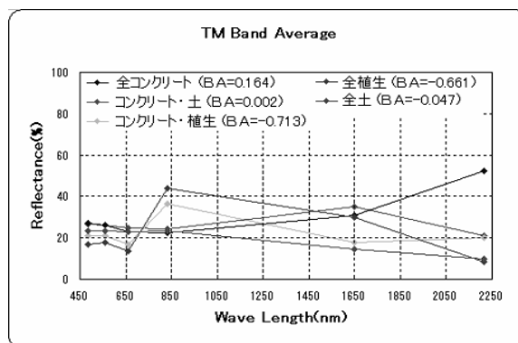
図-2 混合率の異なる地被物の分光反射パターン
