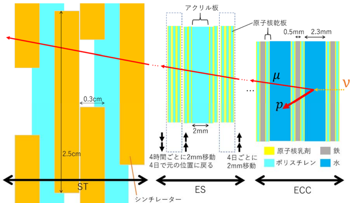
図3 : NINJA 検出器の断面図。ECC は原子核乾板 2 枚で鉄板 1 枚を挟んだユニットと水のサンドイッチ構造になっています。ES は原子核乾板 4 枚とアクリル板を使用した固定壁が真ん中にあり、4 日毎・4 時間毎に 2mm 駆動する駆動壁で構成されます。3 枚の壁の位置関係を元にミュー( \mu )粒子に 4 時間の時間情報をつけます。次に ST はシンチレーター4 層を 1/3 \cdot 1/6 だけズラした構成で、ミュー粒子が貫通して光ったシンチレーターの組み合わせで約 2mm の位置情報・10 ナノ秒ほどの時間情報をつけます。
