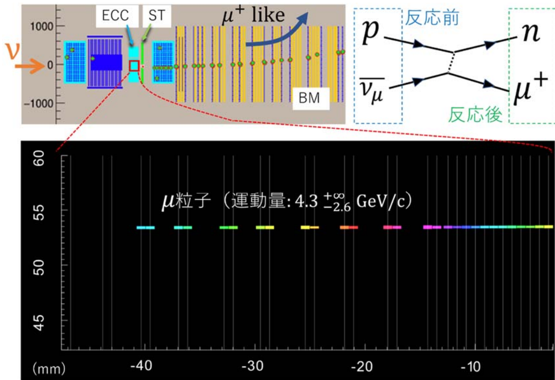
図6：NINJA 実験の解析で検出したニュートリノ反応。反応点からミュー( \mu )粒子が放出されています。 \mu 粒子は複合解析によって下流のBaby MINDにて同定され、磁場による曲がり具合からプラスの電荷を持っています。従って、右上の様式で表されるような、反ニュートリノ( \bar{\nu}_\mu )が陽子(p)と反応し、 \mu^+ 粒子と中性子(n)が生成した反応だと考えられます。中性子は電荷がゼロなので、原子核乾板に信号を残さず、 \mu 粒子の信号のみが写ります。
